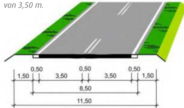
Abb.: Auszug aus den Richtlinien zur Anlage von Landstraßen RAL 2012
